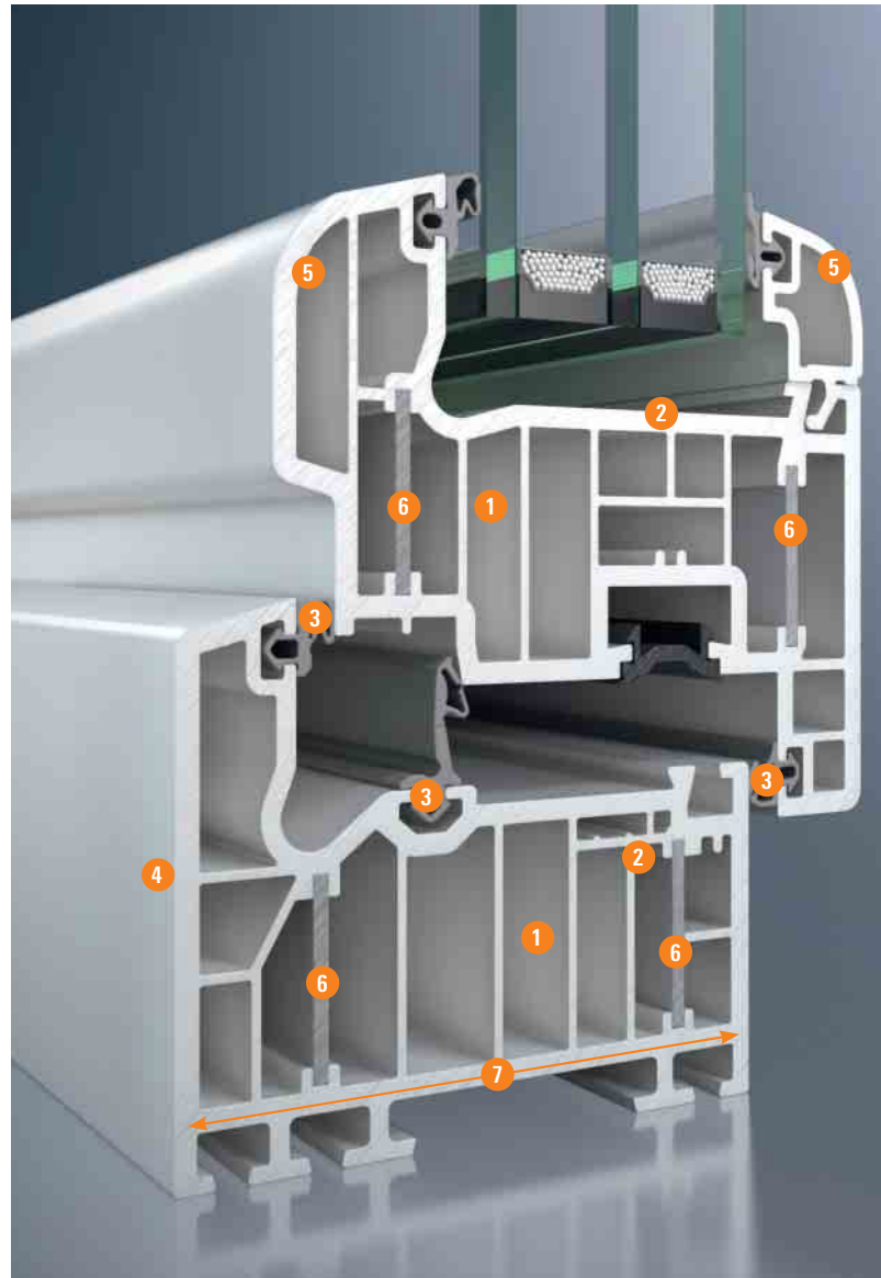
Thermo 8-Fensterprofilsystem
